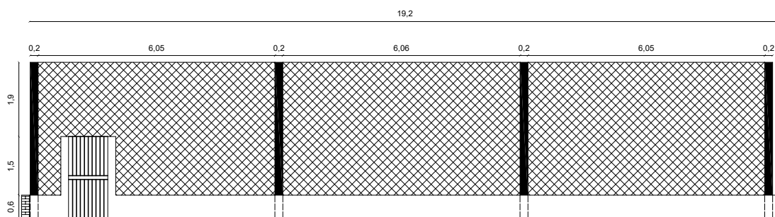
02 VISTA FRONTAL ESCALA 1/100
