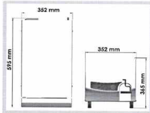
AUTOCLAVE ALT 21L
