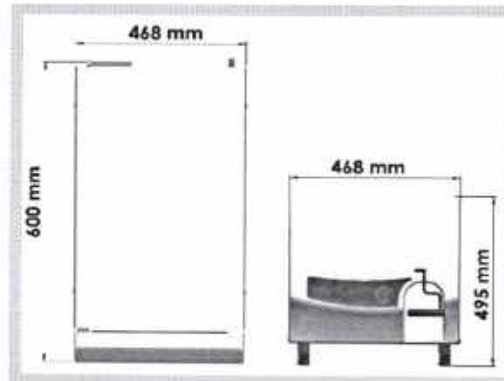
AUTOCLAVE ALT 65L
