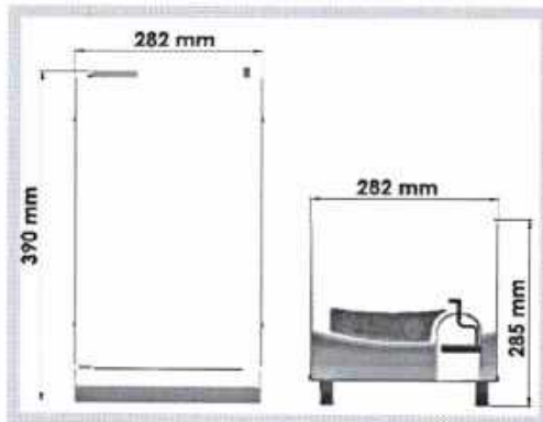
AUTOCLAVE ALT 12L
