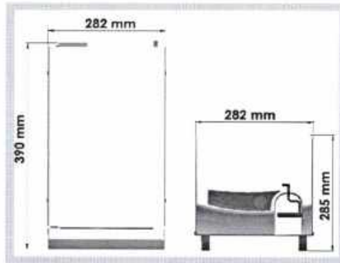
AUTOCLAVE ALT 7L
