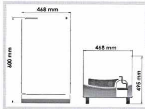
AUTOCLAVE ALT 30L
