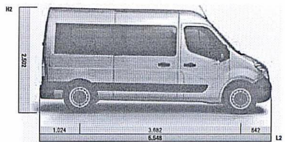
L2H2 STANDARD / ESCOLAR: CHASSI MÉDIO
